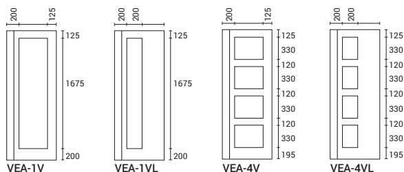
VEA VIDRO EMBUTIDO ALTO
