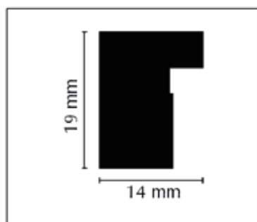
Moldura Lisa a Sobrepor
