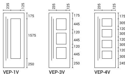
VEP VIDRO EMBUTIDO PARALELO
