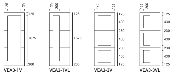
VEA3 VIDRO EMBUTIDO ALTO 3
